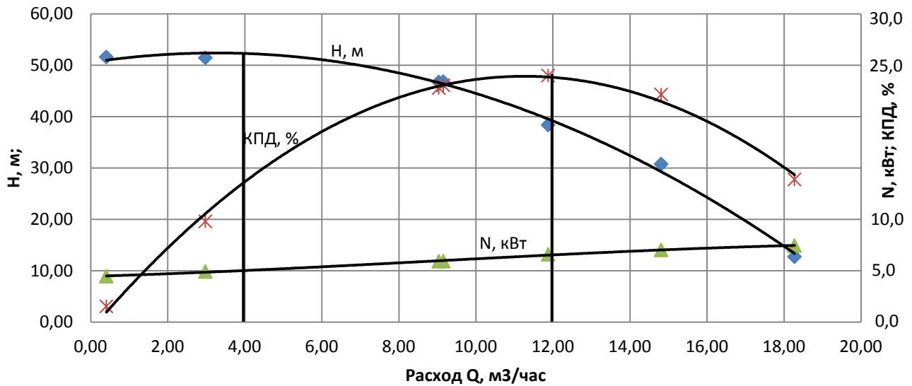
Рабочие характеристики насоса ЦМГ-М 6,3/50 при n=2950 об/мин
