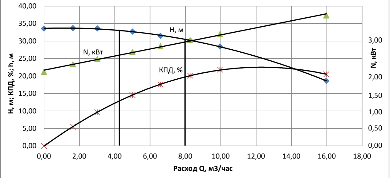
Рабочие характеристики насоса ЦМГ-М 6,3/32 при n=2950 об/мин
