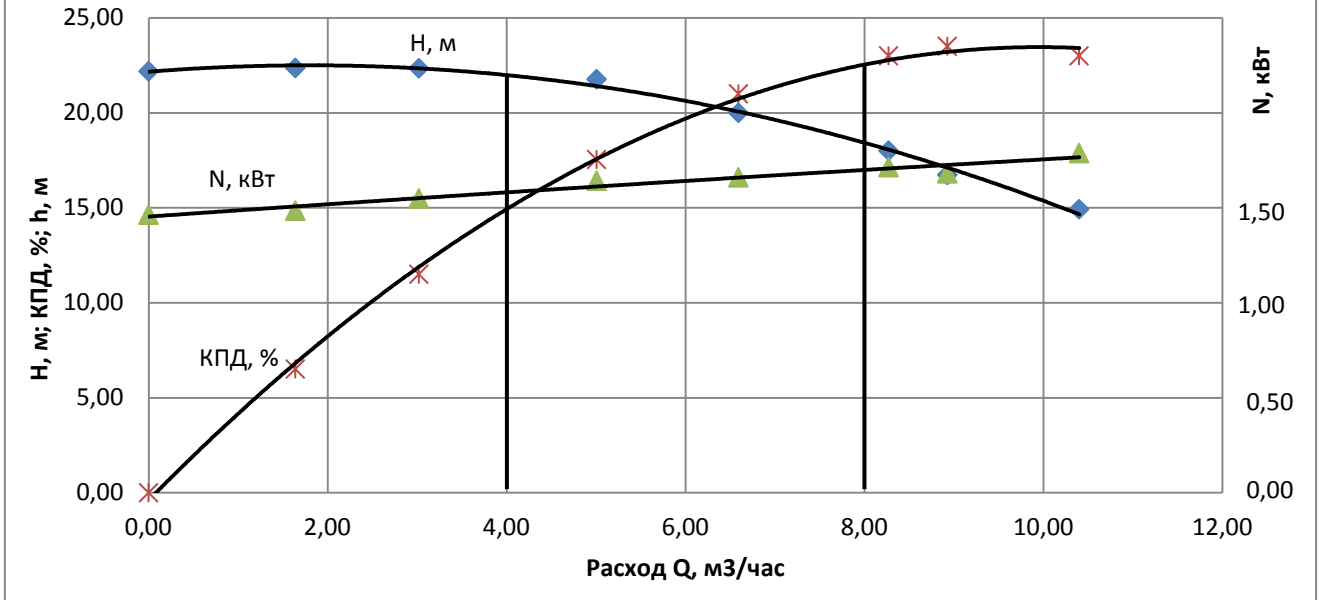
Рабочие характеристики насоса ЦМГ-М 6,3/20 при n=2950 об/мин
