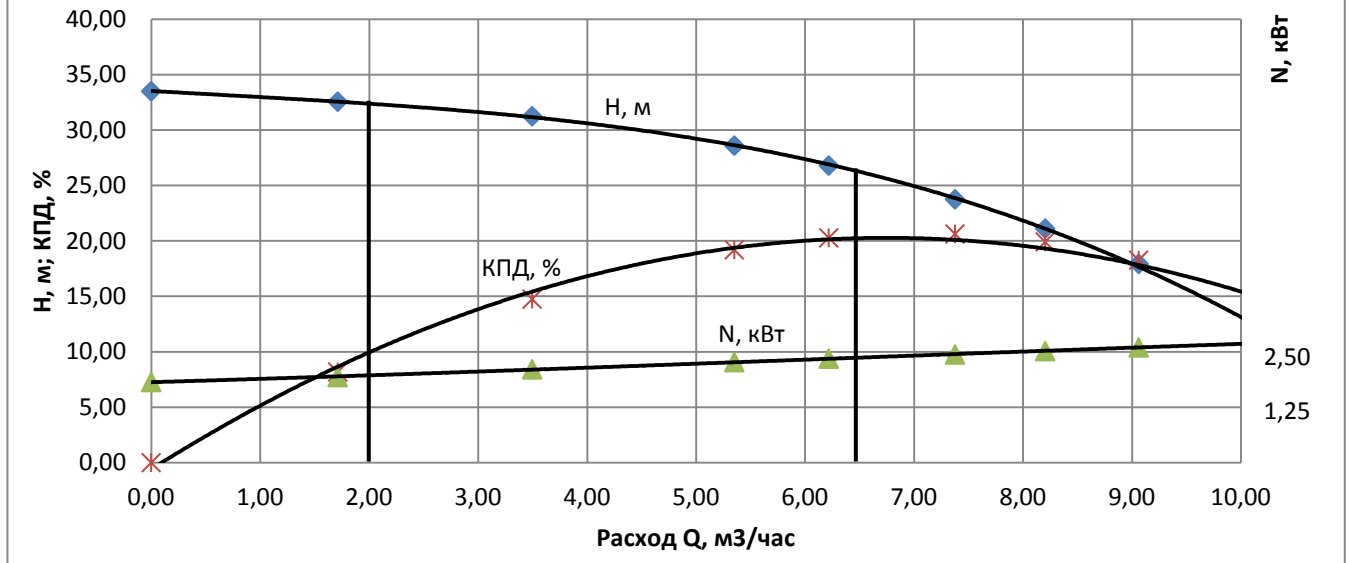
Рабочие характеристики насоса ЦМГ-М 3,2/32 при n=2950 об/мин
