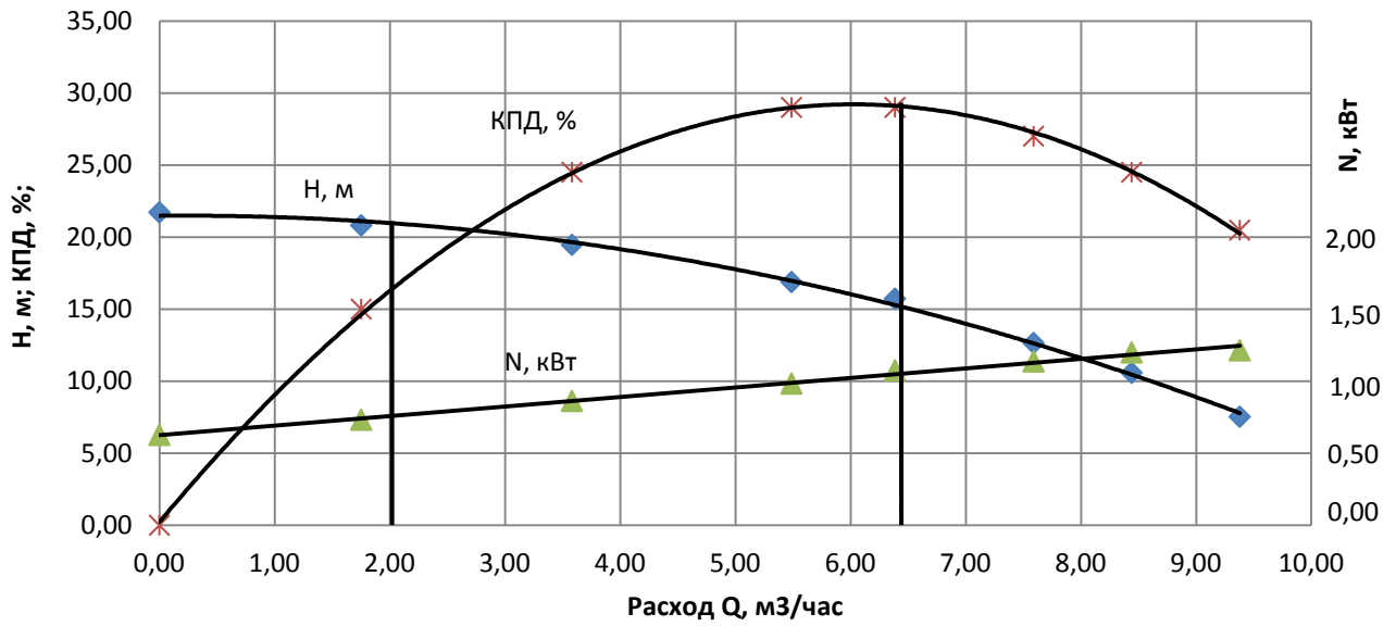
Рабочие характеристики насоса ЦМГ-М 3,2/20 при n=2950 об/мин
