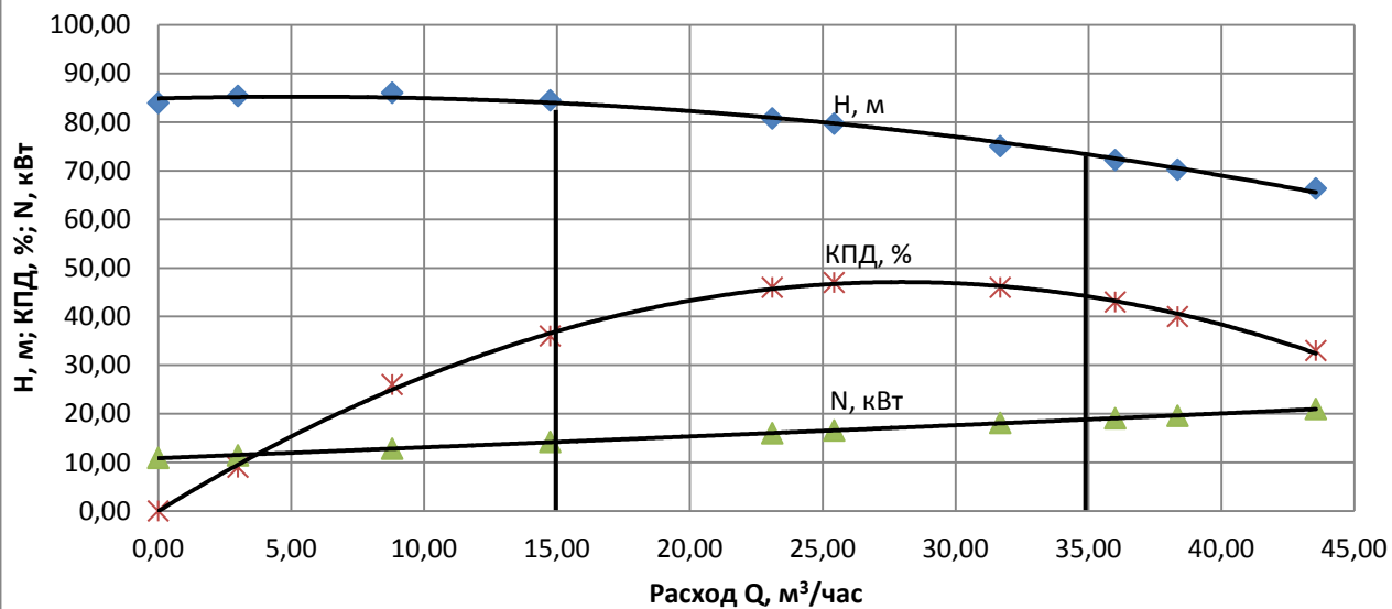
Рабочие характеристики насоса ЦМГ-М 25/80 при n=2950 об/мин
