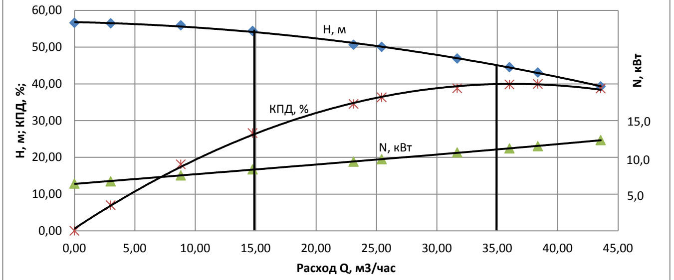
Рабочие характеристики насоса ЦМГ-М 25/50 при n=2950 об/мин
