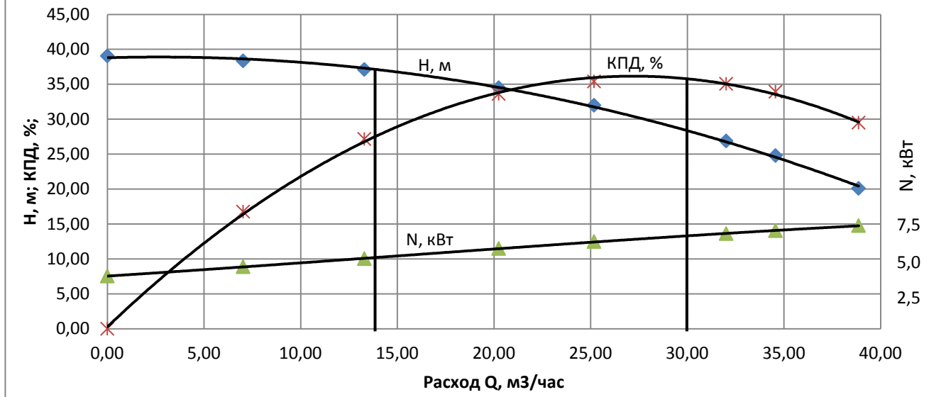
Рабочие характеристики насоса ЦМГ-М 25/32 при n=2950 об/мин
