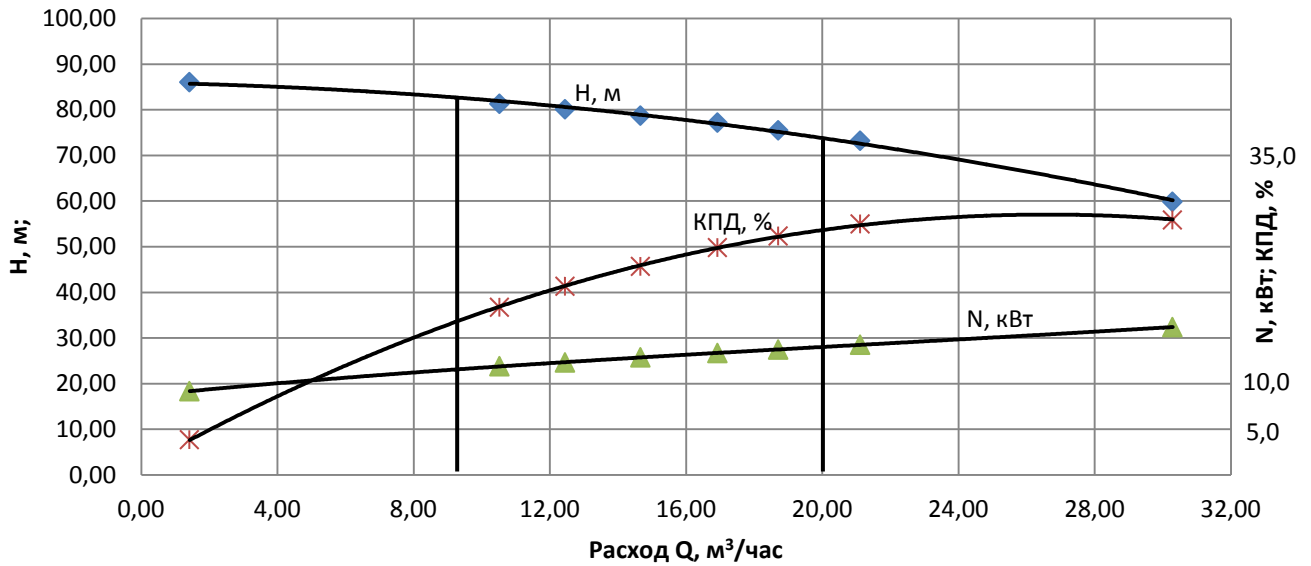
Рабочие характеристики насоса ЦМГ-М 12,5/80 при n=2950 об/мин
