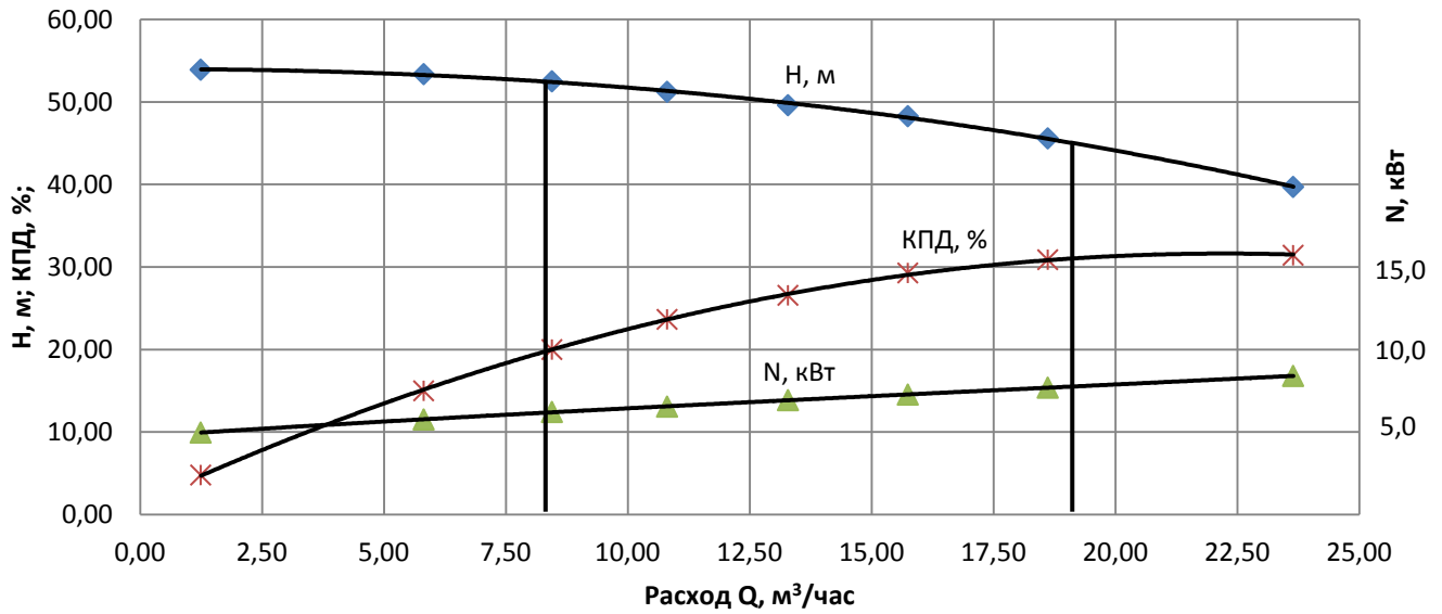
Рабочие характеристики насоса ЦМГ-М 12,5/50 при n=2950 об/мин
