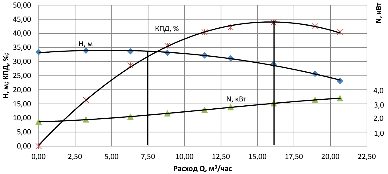
Рабочие характеристики насоса ЦМГ-М 12,5/32 при n=2950 об/мин
